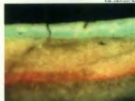
Figura 6 - Estrati-gráfica da aniseeds retirada do manto azul claro, 20x (vide Imagem 2)
