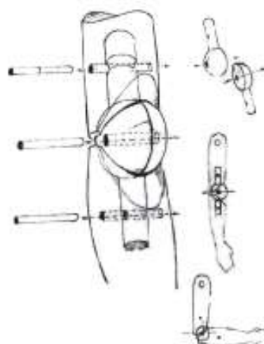
FIGURA 6 - Articulação esfera bipartida
