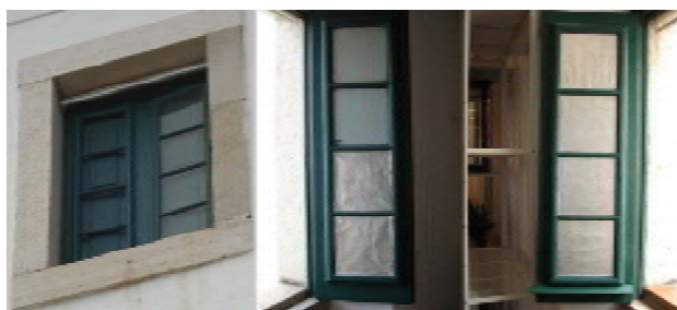
Figura 3: Caixilhos originais da sala, teste com diferentes tipos de películas de materiais opacos e caixilho pronto com aplicação de Tyvek, para reduzir carga térmica
